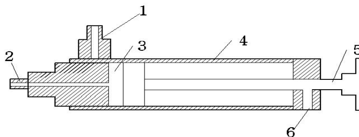
图1 高负压瓦斯采取器
